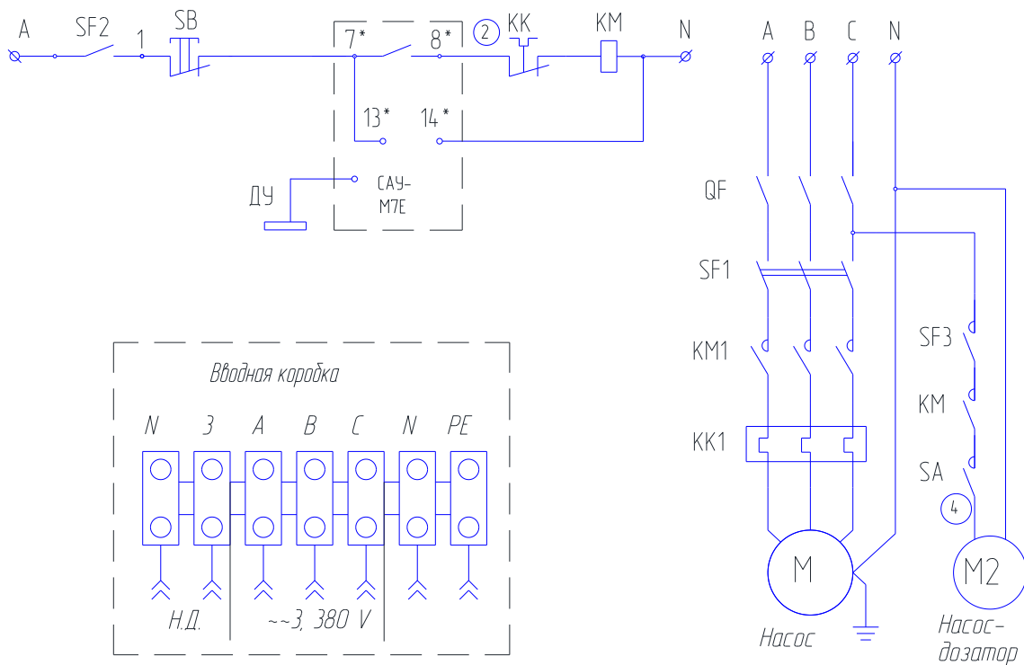
Рис. 2. Схема принципиальная
