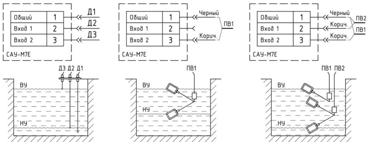
Рис. 4. Монтаж датчиков уровня.
